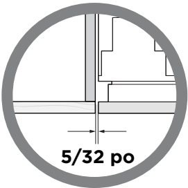
DÉGAGEMENT VERTICAL À PARTIR DU CÔTÉ DU PANNEAU DE PORTE
