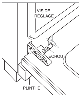
Alignement de la porte
