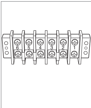
Conexión eléctrica
