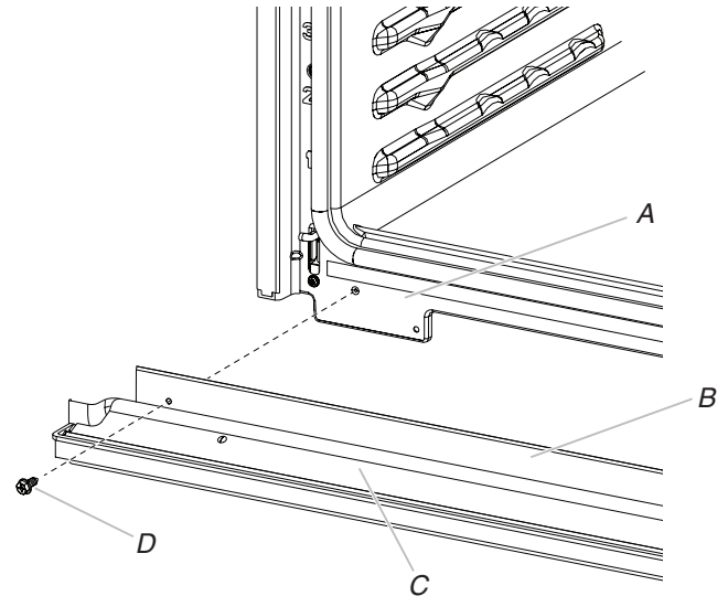
A. Châssis du four B. Onglet de l'évent C. Évent du four D. Vis no 8-18 x 3/8" (9,5 mm)
