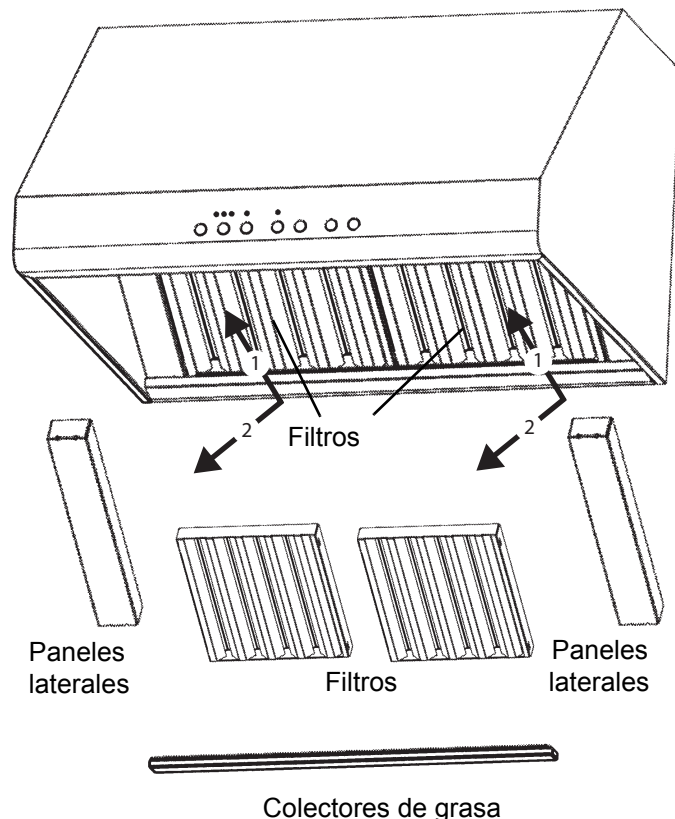
Figura 3: La campana y sus piezas
