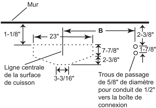
Vue en plan de l'entaille de l'armoire
