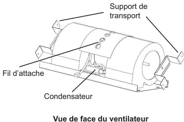
Figure 13 : Vue de face du ventilateur
