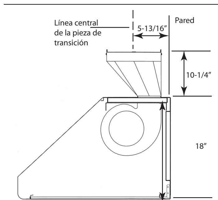
Figura 8: Línea central de la pieza de transición para la salida vertical
