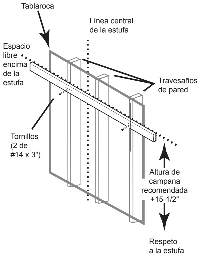
Figura 4: Montaje del soporte de madera
