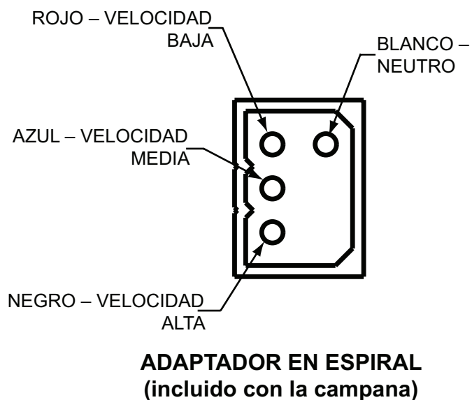
Figura 21: Cableado de la campana con un ventilador en línea
