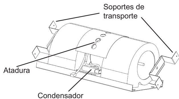
Vista de frente del ventilador
