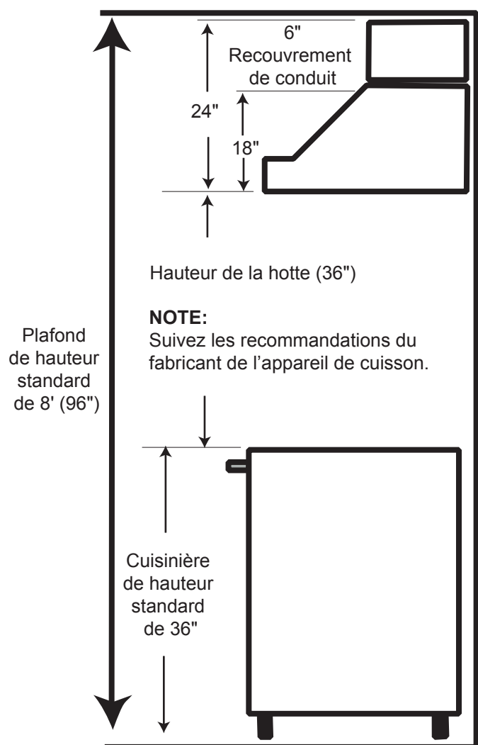
Figure 3 : Installation caractéristique de la hotte
