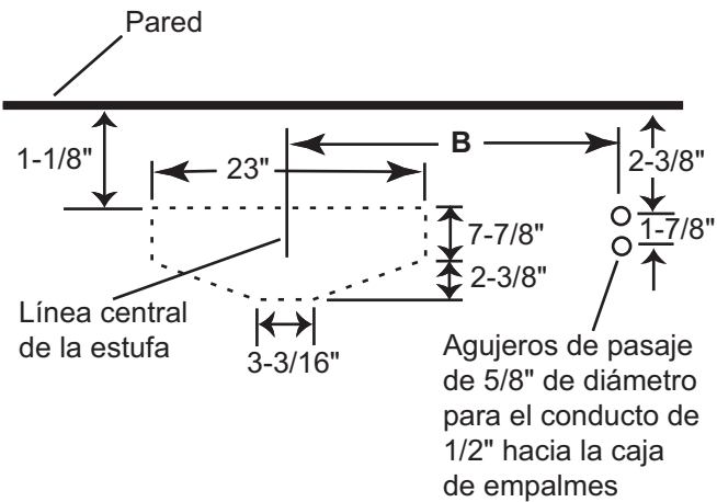
Vista en planta del corte del armario
