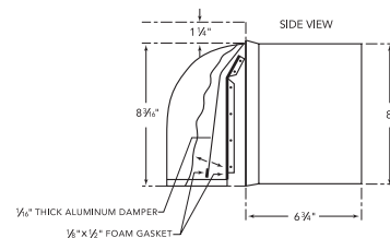
10-Inch Wall Cap – WC10
