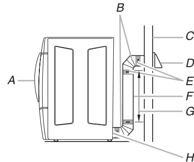
A. Secadora B. Codo C. Pared D. Capota de ventilación E. Abrazaderas
