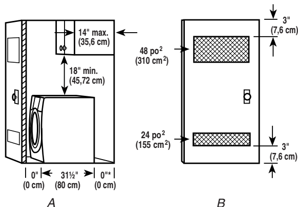
A. Vue latérale - placard ou endroit exigu B. Porte de placard avec orifices d'entrée d'air *Évacuation par le côté ou par le fond
