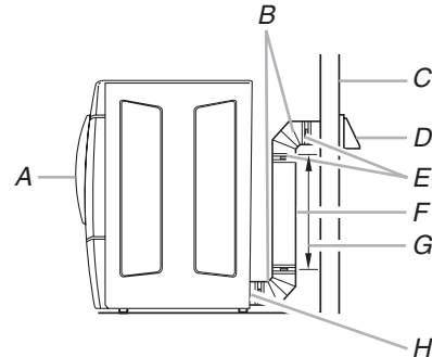
A. Sècheuse B. Coude C. Mur D. Clapet de décharge E. Brides
