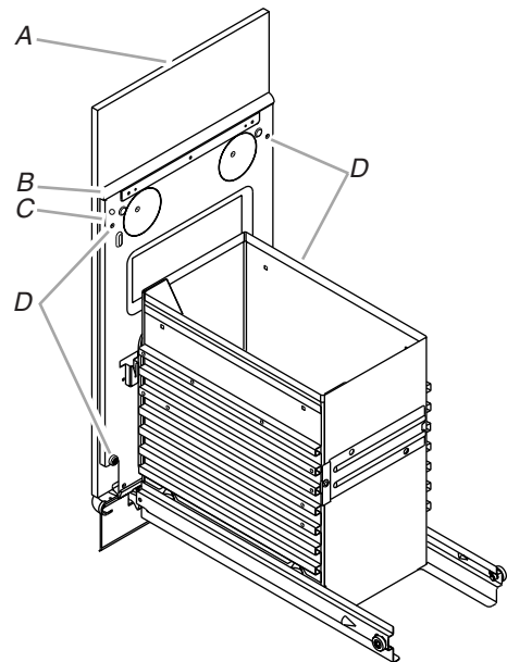
A. Panneau personnalisé B. Quart-de-rond de 15" x 1/2" C. Façade du tiroir D. Position des quatre vis à bois n° 8 x 1"
