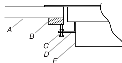
A. Plan de travail B. Cale en bois C. Vis de retenue D. Brides de retenue E. Boîte des brûleurs
