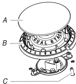
A. Chapeau B. Répartiteur C. Électrode
