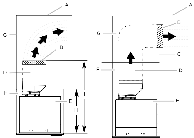
A. Plafond B. Cache-conduit C. Soffite D. Évent de 6" (15,2 cm) E. Hotte de cuisinière
