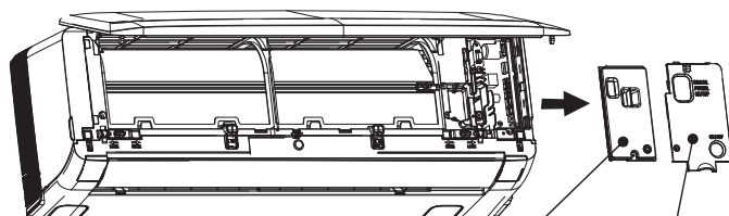
couvercle de boîte électrique couvercle du câblage
