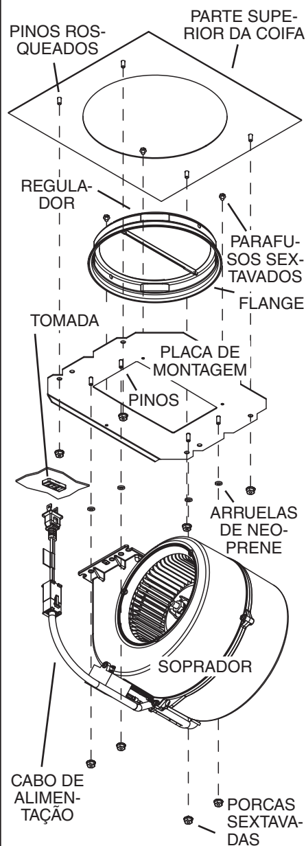
Configuração do ventilador usando a placa de montagem 020971-000
