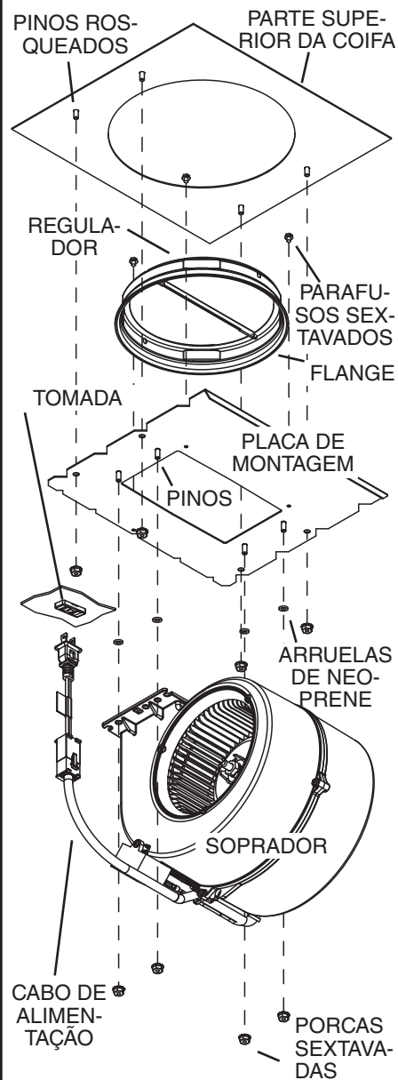
Configuração do ventilador usando a placa de montagem 020972-000 ou 050722-000
