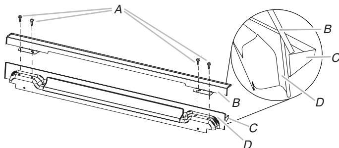
A. Vis n° 8-18 x ¼" B. Déflecteur pour tiroir-réchaud C. Évent D. Vis n° 8-18 x 3/8"
