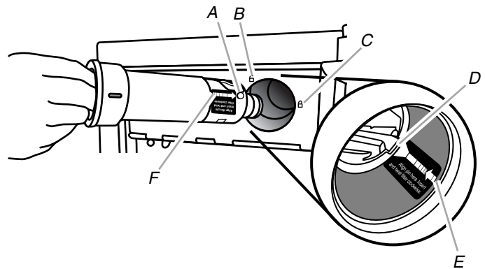
A. Espiga de alineamiento B. Símbolo de desbloqueo C. Símbolo de bloqueo D. Muesca recortada dentro del alojamiento del control E. Flecha apuntando a la muesca recortada F. Flecha apuntando a la espiga de alineamiento
