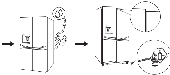
4 Conexión del suministro de agua y del conducto de agua
