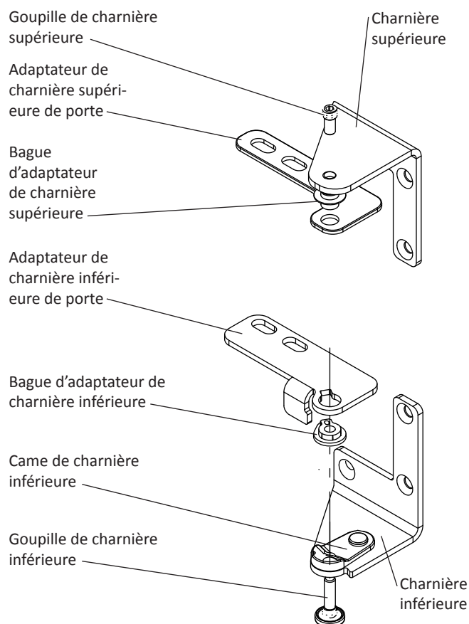
Figure 14 Charnières montrées du côté droit
