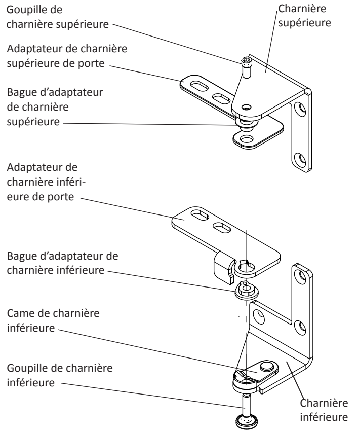
Figure 12 Charnière montrées du côté droit
