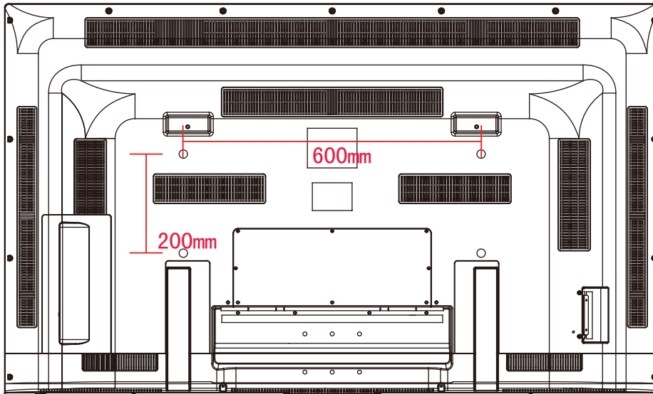
Dimensions pour des trous de montage
