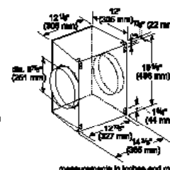
VTI1010D—1000 CFM
