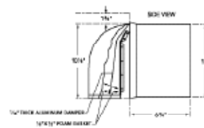
Wall Cap—WC10
