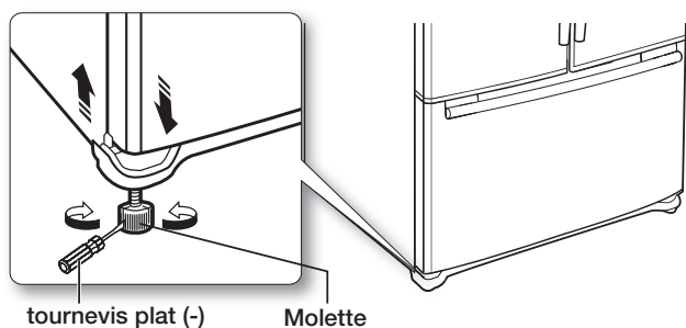
tournevis plat (-)
