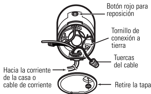
Fondo del triturador (campana extremo)
