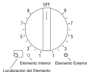
Figura 5: Perilla de control de un elemento doble
