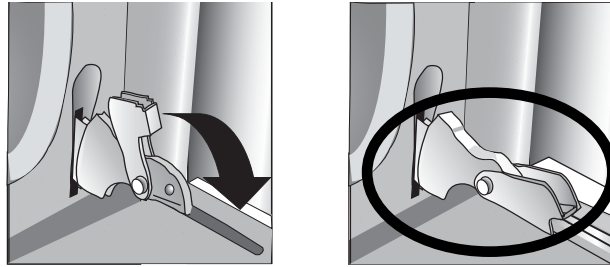
Figure 10 : Positions de charnières
