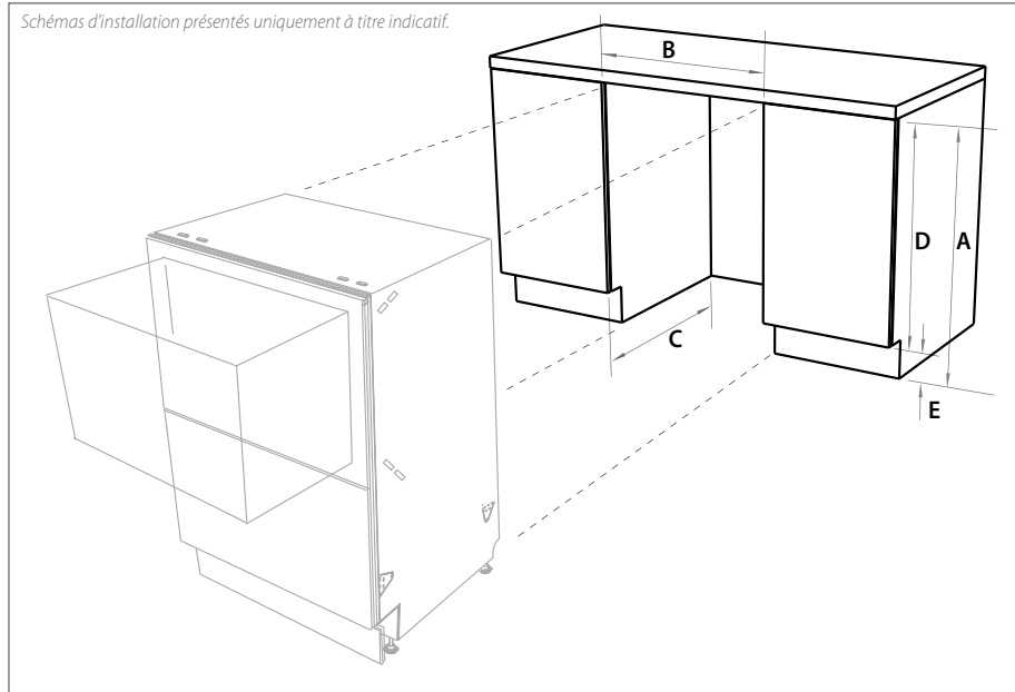
Dimensions des armoires (pouces [mm])
