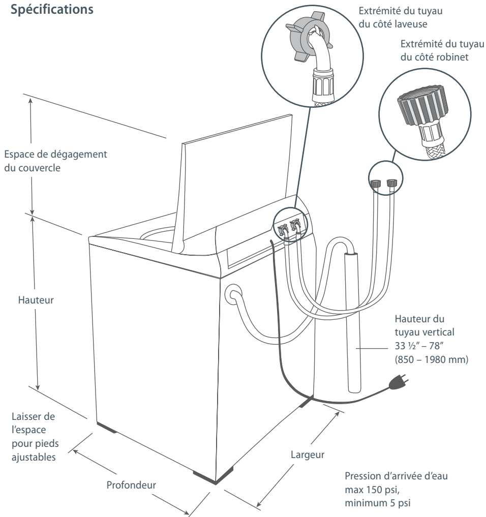
Fig.1 Dimensions de la laveuse et raccords
