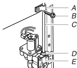
A. Bride du tube B. Vis de bride de tube C. Tube en cuivre D. Écrou de compression E. Valve d'entrée d'eau
