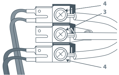
Dibujo 24 Conectar los cables
