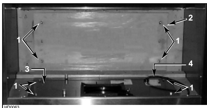
1. Tuercas 3. Placa ventilador a detrás de la campana 2. Placa sobre encima de la campana 4. Cubierta de la caja de cableado
