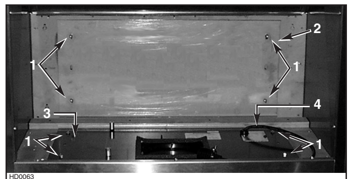
1. Écrous dentelés 2. Plaque sur le dessus de la hotte 3. Plaque ventilateur à l'arrière de la hotte 4. Couvercle du boîtier électrique
