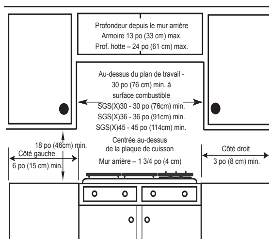
Figure 1 : Dimensions d'installation (depuis les bords de la plaque de cuisson)
