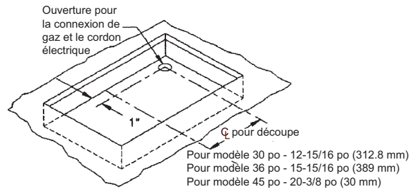
Figure 5 : Zone de la boîte brute
