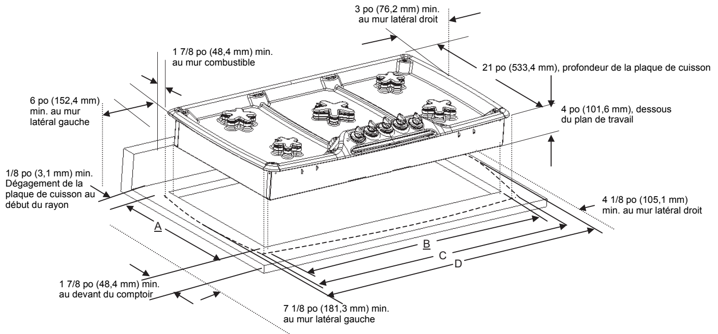
Figure 2 : Dimensions de découpe
