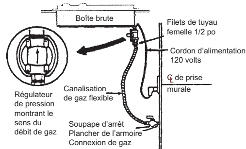
Figure 6 : Emplacement du gaz et de l'électricité
